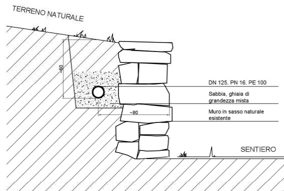
Sezione tipo A-A
